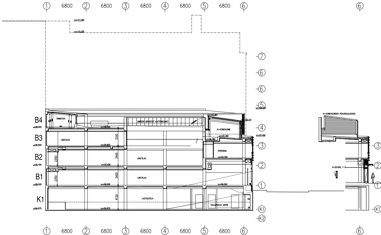
Leikkaus
