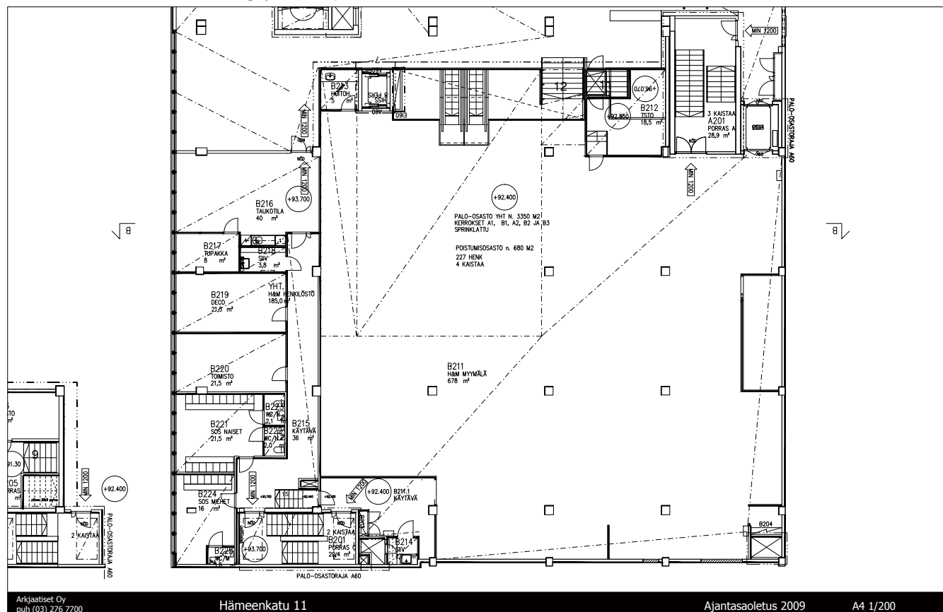
Pohjapiirustus, osa2
