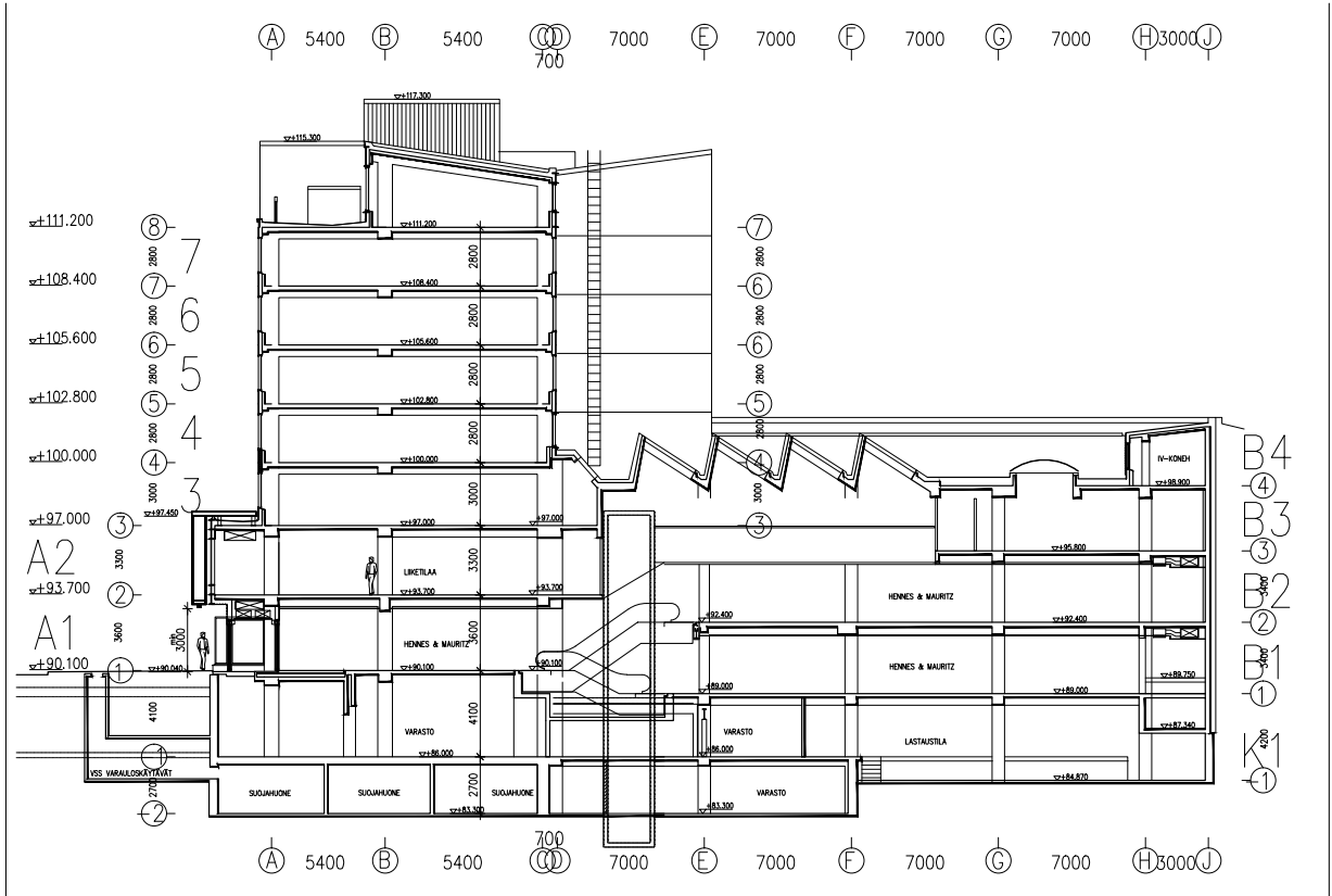
Leikkaus
