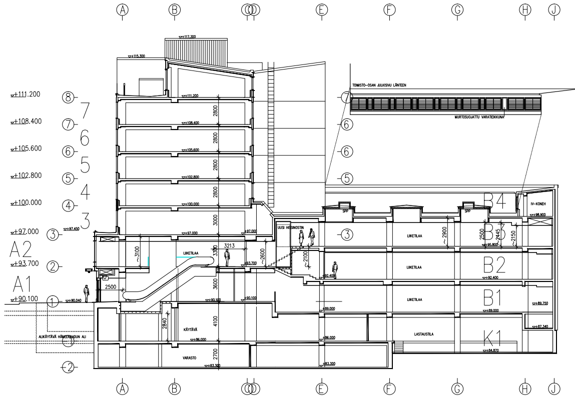
Leikkaus
