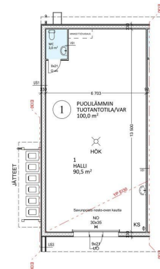
TILA 1
