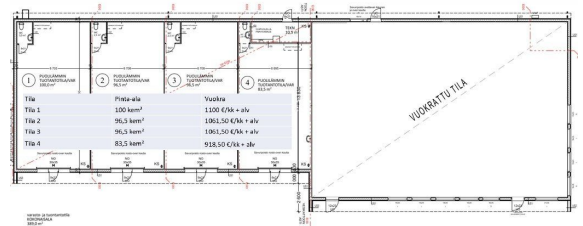
Pohjakuva
