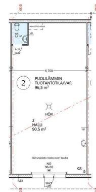
TILA 2
