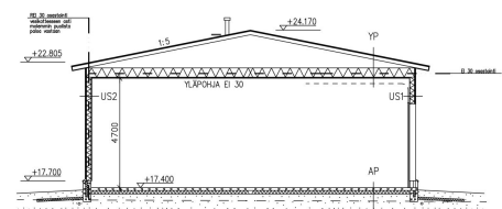
LEIKKAUS A-A
