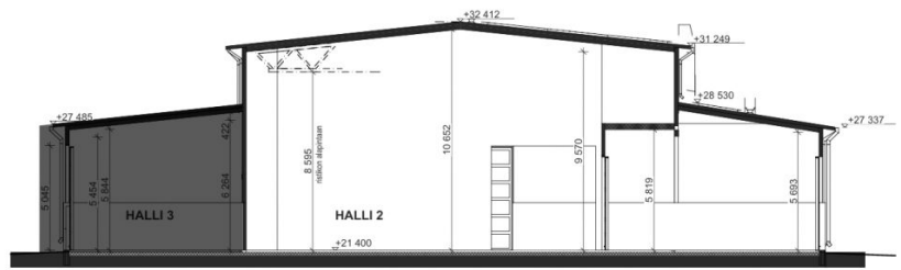
Leikkaus A-A
