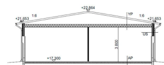
Leikkaus A-A 1:100
