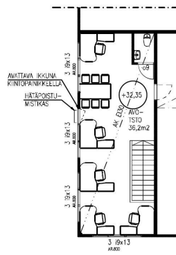
POHJAPIIRUSTUS 2.KRS 1:100
