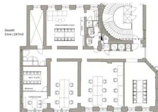
Toimistotila 3. krs 247m 2
