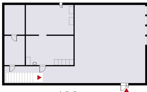
kellarikerros
