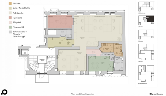
Toimisto A5 Pohjapiirustus, ei mittakaavassa Huoneistoa 119,5m 2
