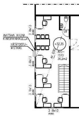
POHJAPIIRUSTUS 2.KRS 1:100
