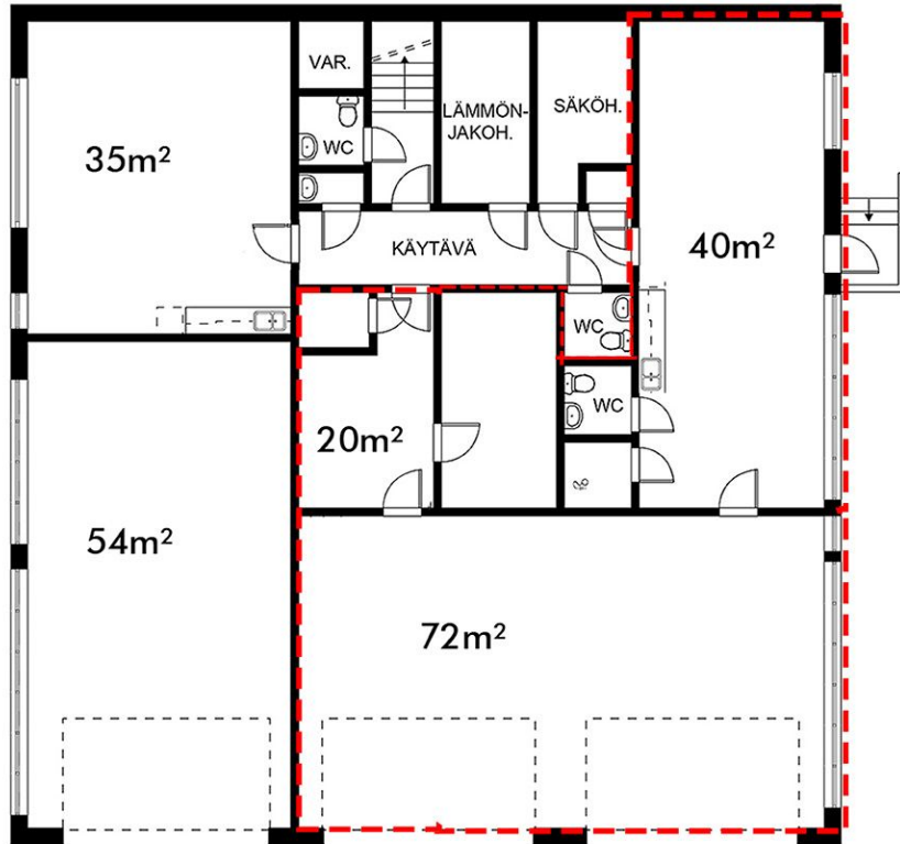
Katutasen pohjakuva
