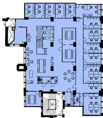
2. KERROS
