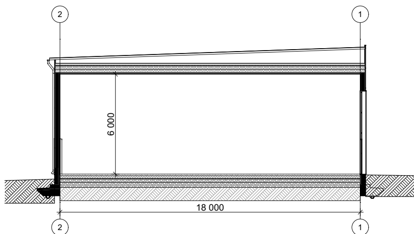
A1 LEIKKAUS
