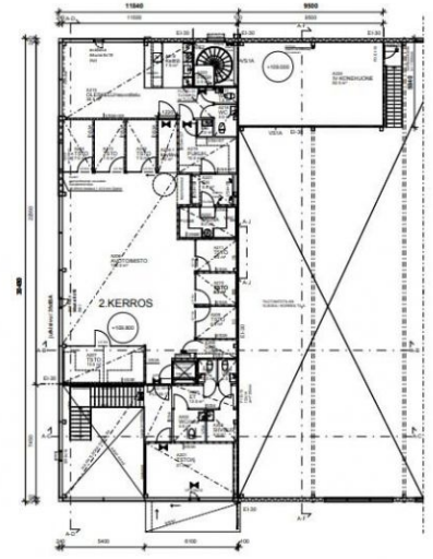
2. KERROS 1:100
