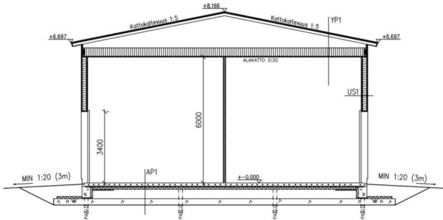
LEIKKAUS A - A:
