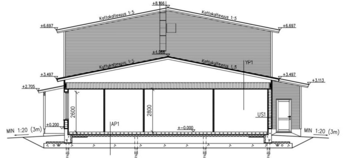
LEIKKAUS B - B:
