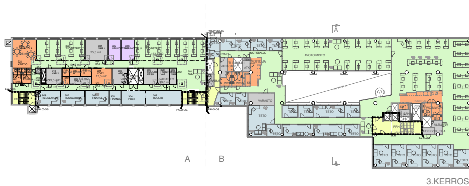
3. KERROS
