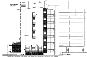
Julkisivu Länteen 1:400
