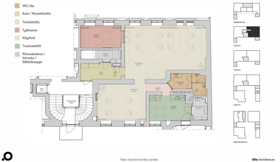
Toimisto A5 Pohjapiirustus, ei mittakaavassa Huoneistoa 119,5m 2
