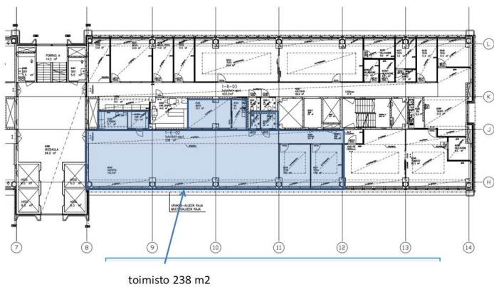
Pohjapiirustus toimisto 238
