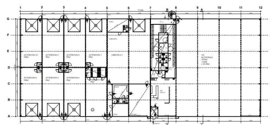
pohja 1.kerros 1:100
