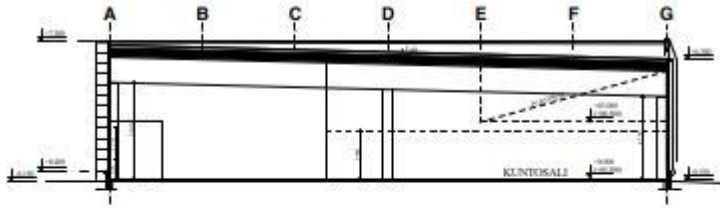
leikkaus A-A 1:100
