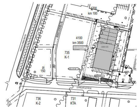
asemapirros 1:500
