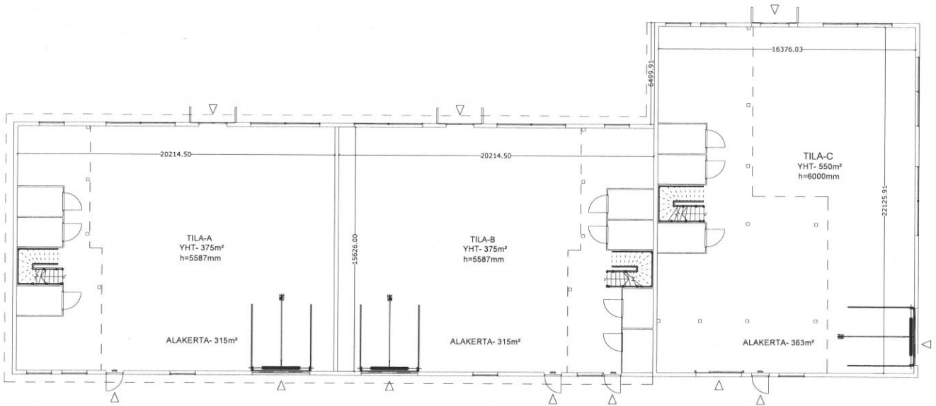
Pohjapiirustus Kerros:1
