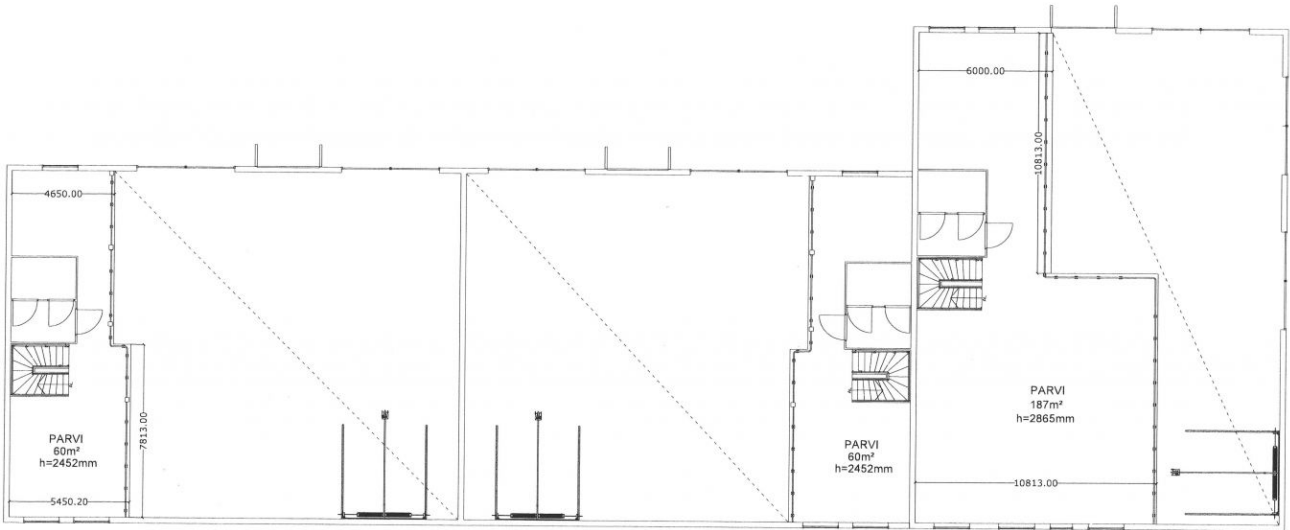
Pohjapiirustus Kerros:2
