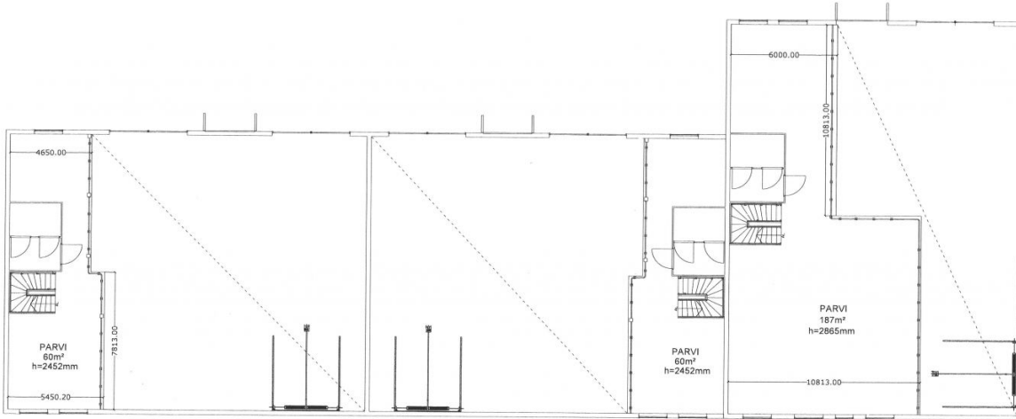
Pohjapiirustus Kerros:2
