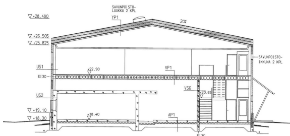
LEIKKAUS A-A
