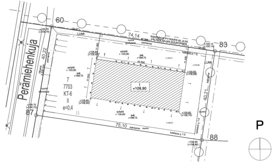
Asemapiirros 1:500
