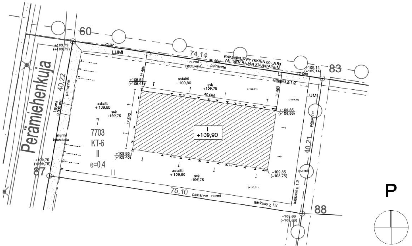
Asemapiirros 1:500
