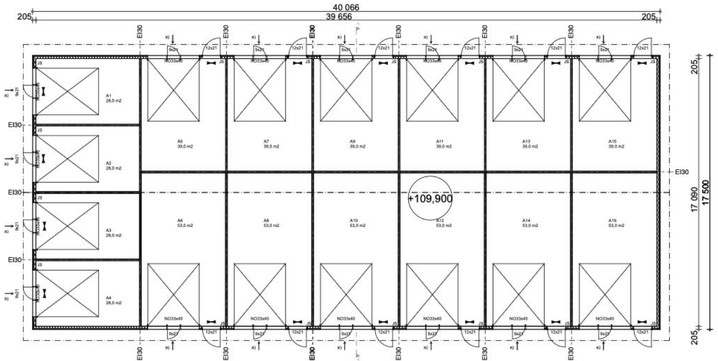
Pohjapiirustus 1:100
