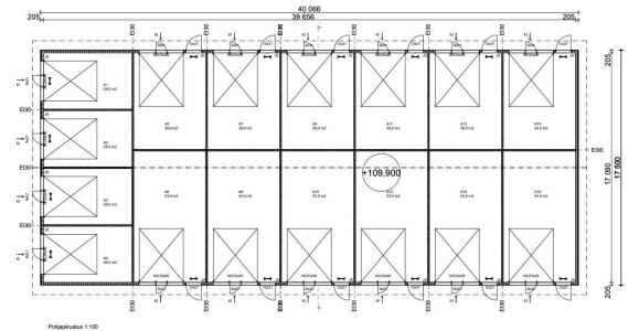
Pohjapiirros 1:100
