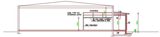
LEIKKAUS A-A 1:100
