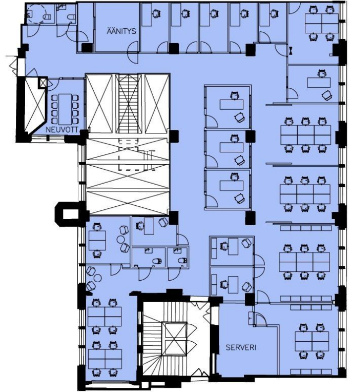
3. KERROS
