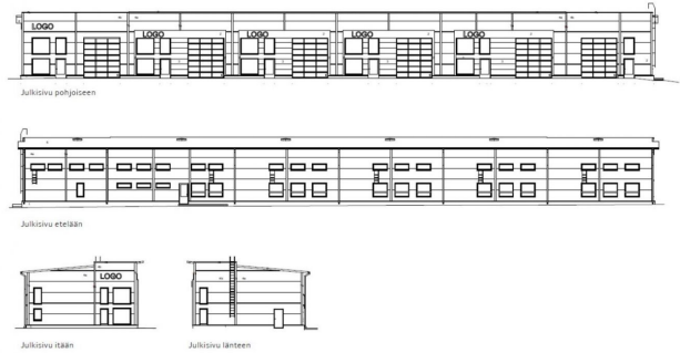
Julkisivut
