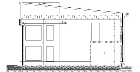
Leikkauskuva
