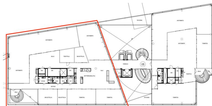
1:150 2. KERROS, POHJA 08.02.2023 arkitehdit
