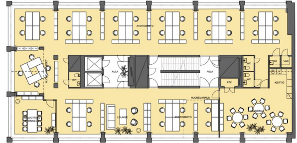
410 m 2 3. KERROS
