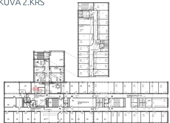
POHJAKUVA 2.KRS
