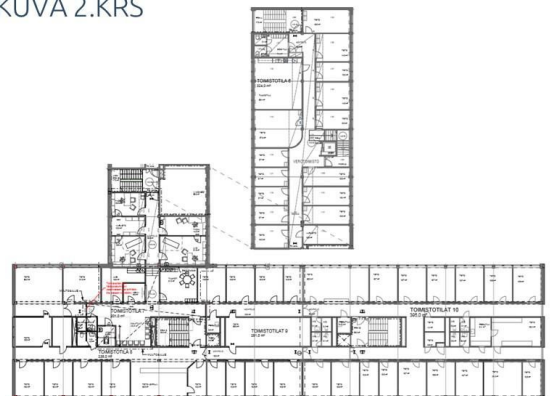
POHJAKUVA 2.KRS
