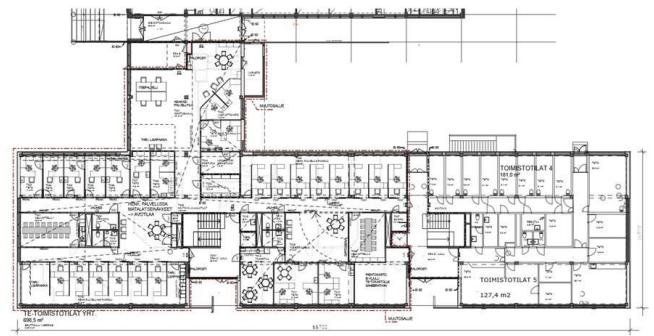
POHJAKUVA 1.KRS (1/2)
