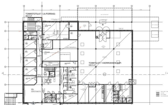
POHJAKUVA 1.KRS (2/2)
