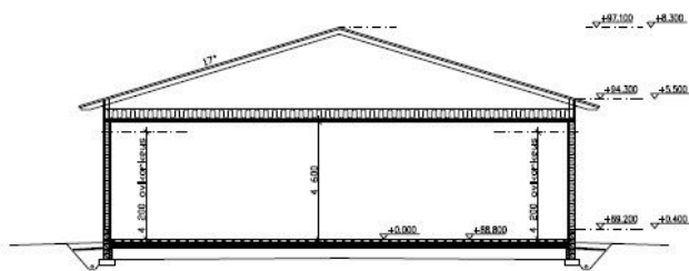
LEIKKAUS A - A
