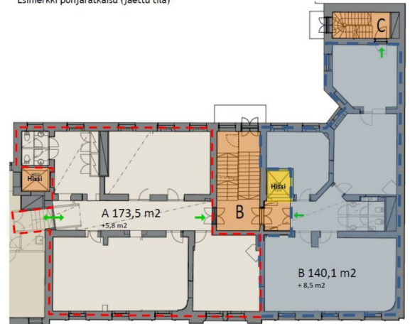
Esimerkki pohjaratkaisu (jaettu tila)
