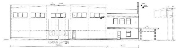
JULKISIVUT MK 1:100
