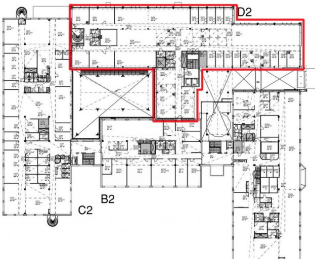
Pohjapiirustus
