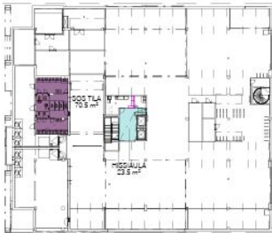
KELLARI
