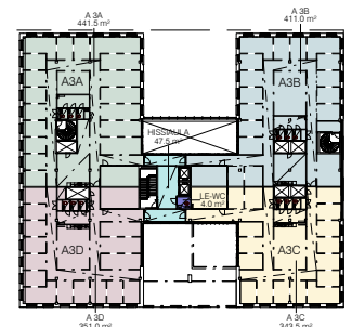
3. KERROS
