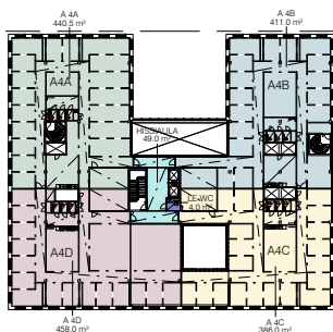
4. KERROS
