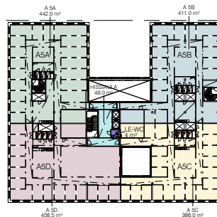
5. KERROS
