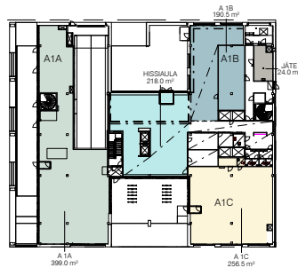
1. KERROS
