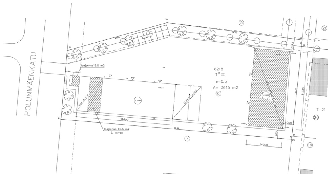
Asemapiirustus, ei mittakaavassa
