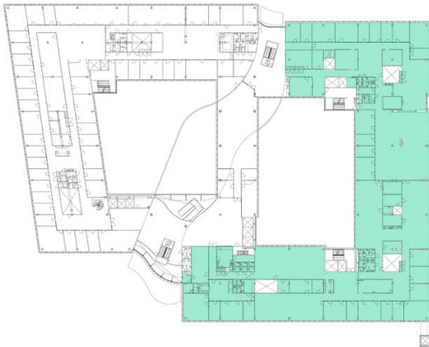
6. KERROS vuokrattava huoneistoala ~ 2175 m 2
