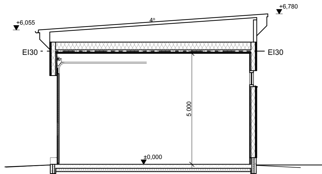
LEIKKAUS A-1 1:100
