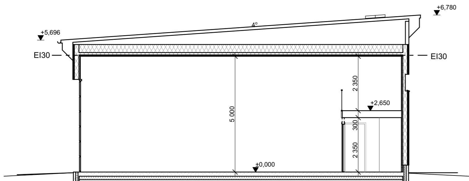
LEIKKAUS A-2 1:100
