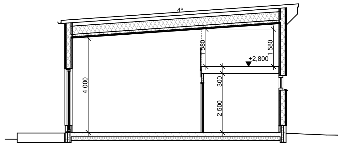
LEIKKAUS B-1 1:100
