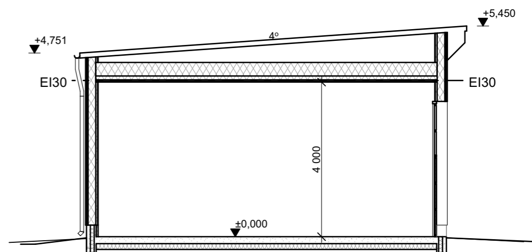
LEIKKAUS B-2 1:100
