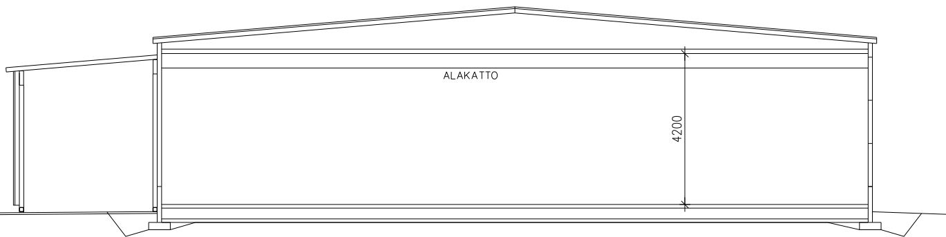
LEIKKAUS A-A
