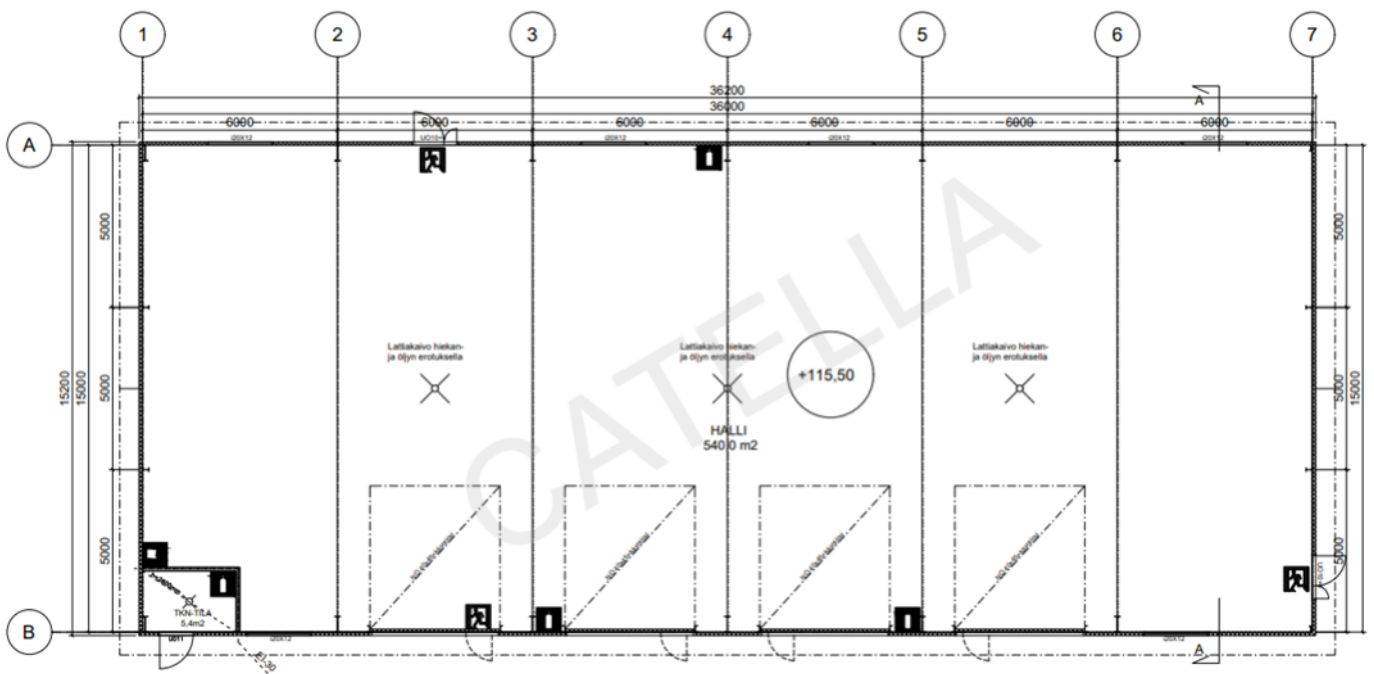
Pohjapiirustus, ei mittakaavassa.
