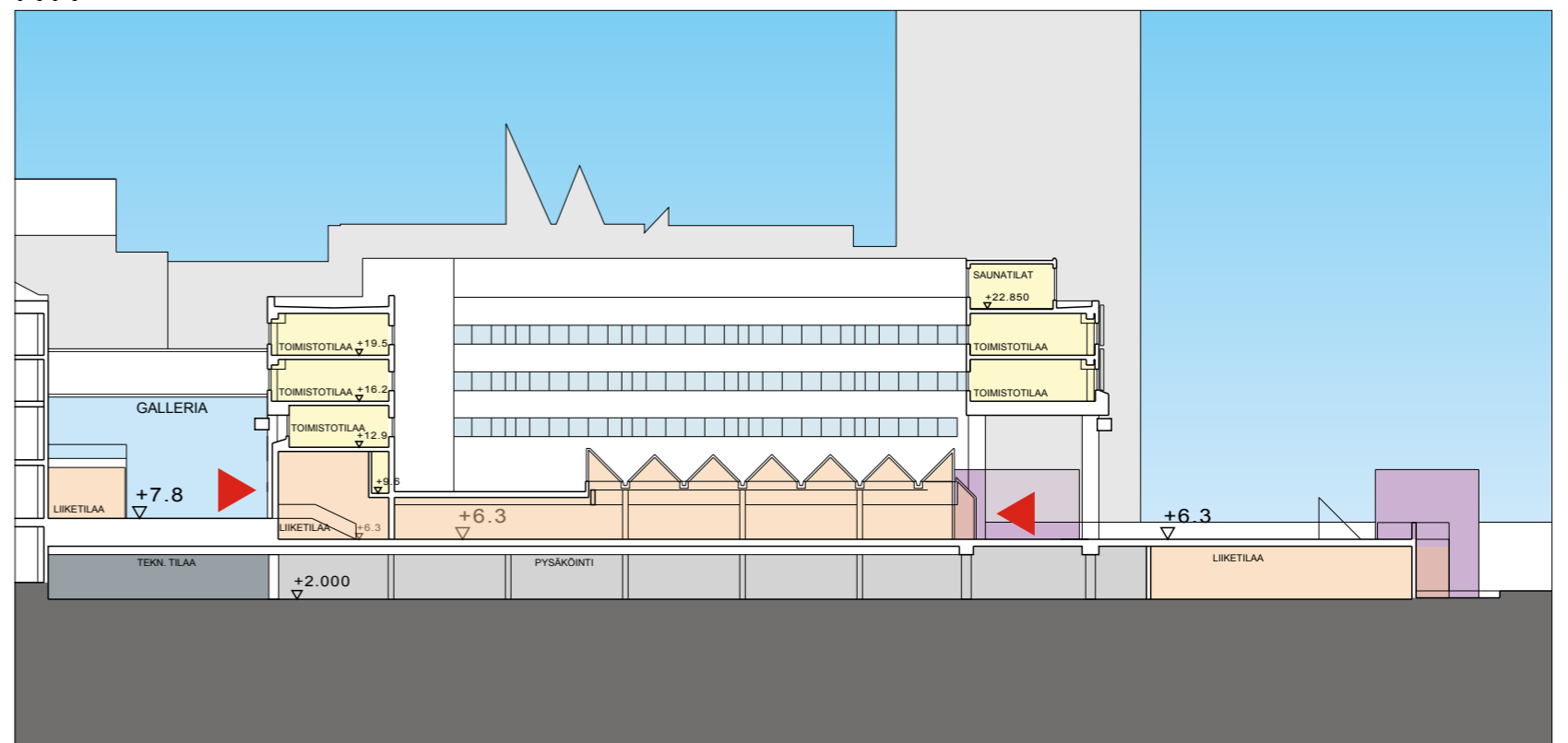
B-B
