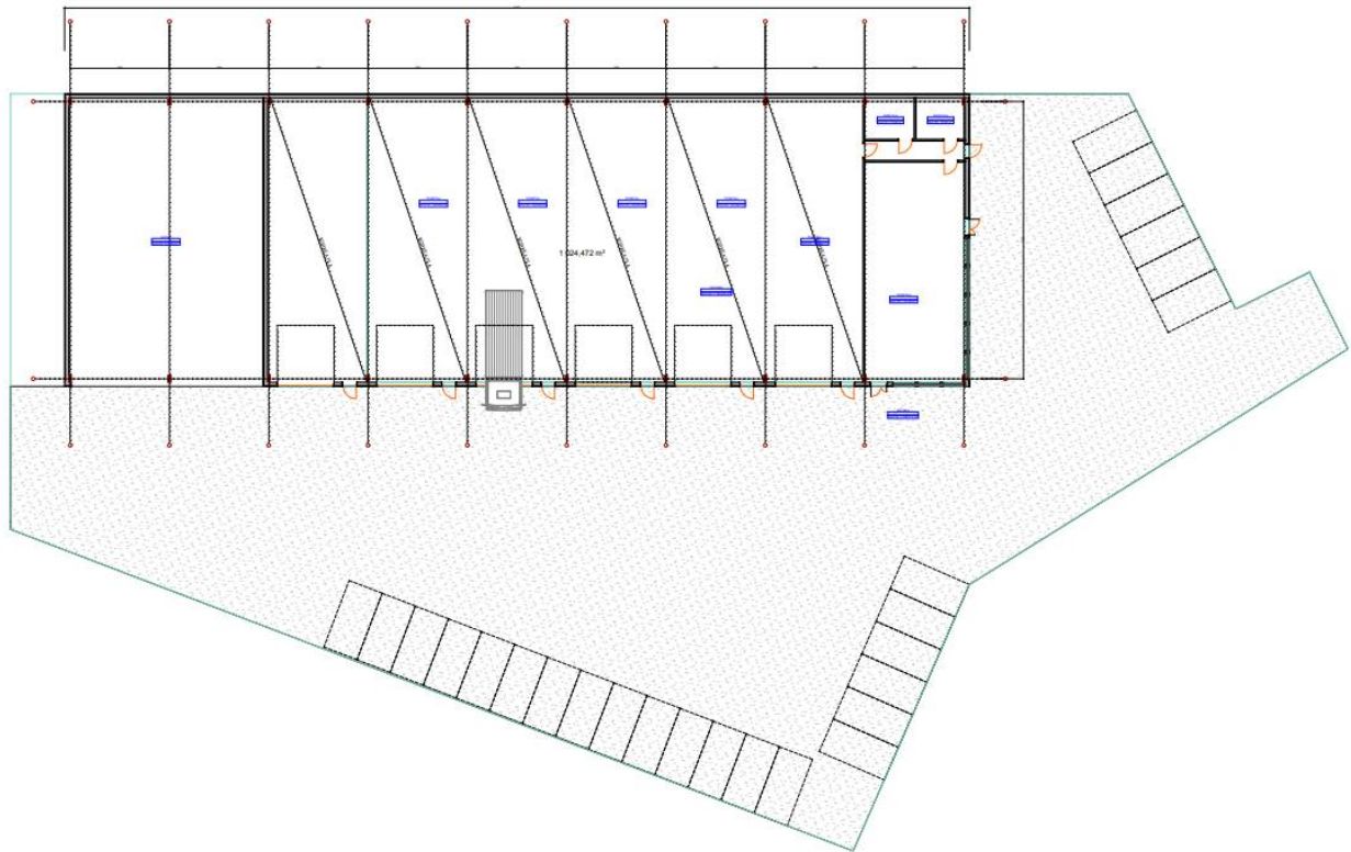
katutasokerros, suuntaa antava, ei mittakaavassa
